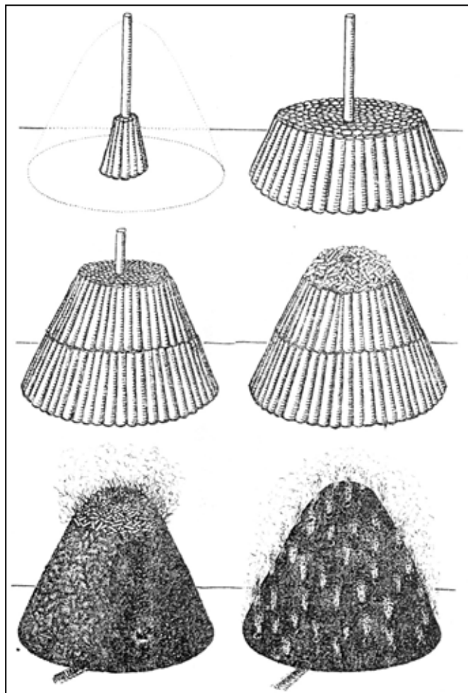
Schéma stavby milíře (nakreslil Josef Dohnal)
